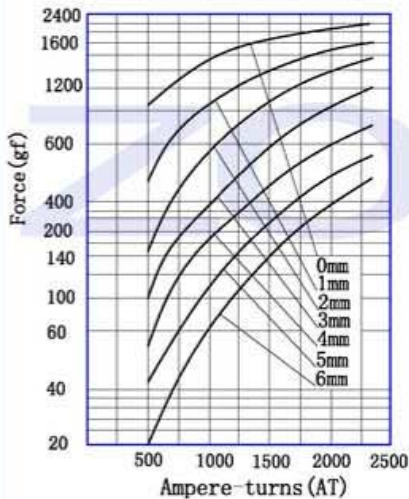
行程/吸引力 STROKE Vs FORCE
